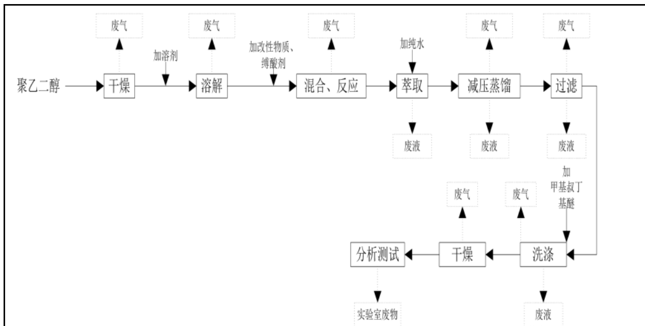
图 2-7 改性聚乙二醇研发工艺流程及产污环节图
