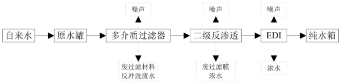
图 2-8 制纯水工艺工艺流程及产污环节图
