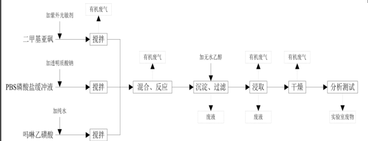
图 2-3 改性透明质酸钠研发工艺流程及产污环节图
