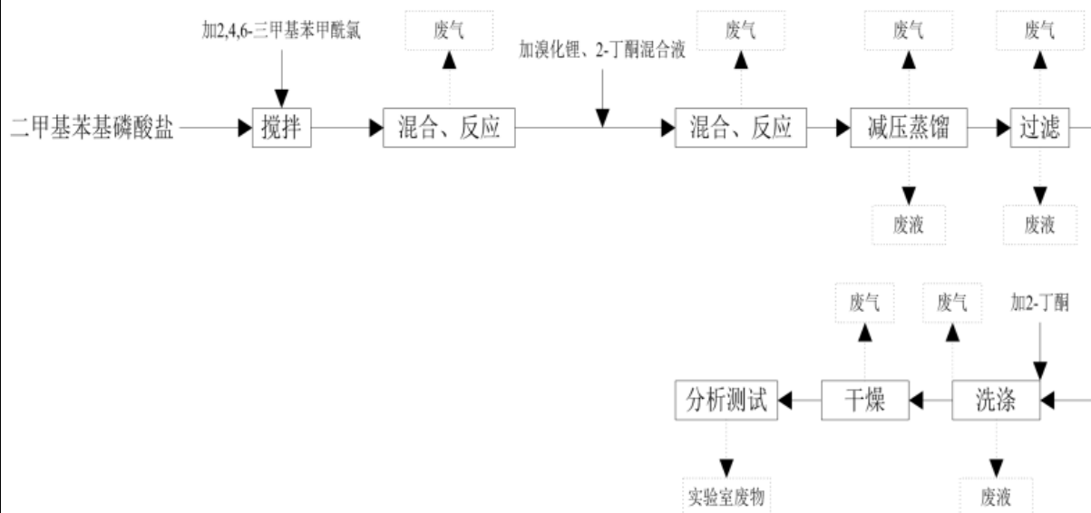
图 2-6 高效紫外光引发剂研发工艺流程及产污环节图
