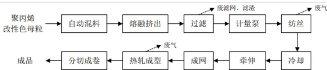
图 2-2 生产工艺及产污流程图
