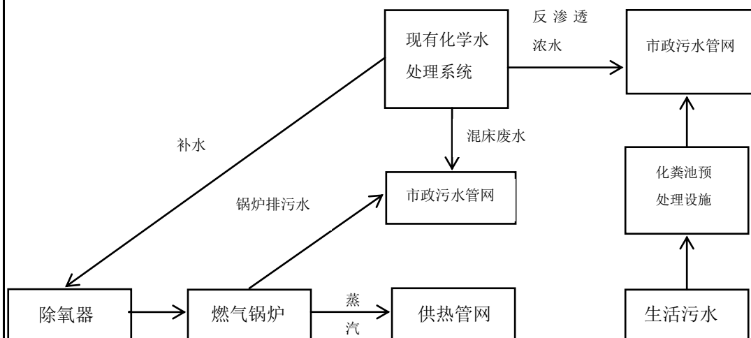
图 2-1 营运期 2 号能源站工艺流程及产污环节示意图
