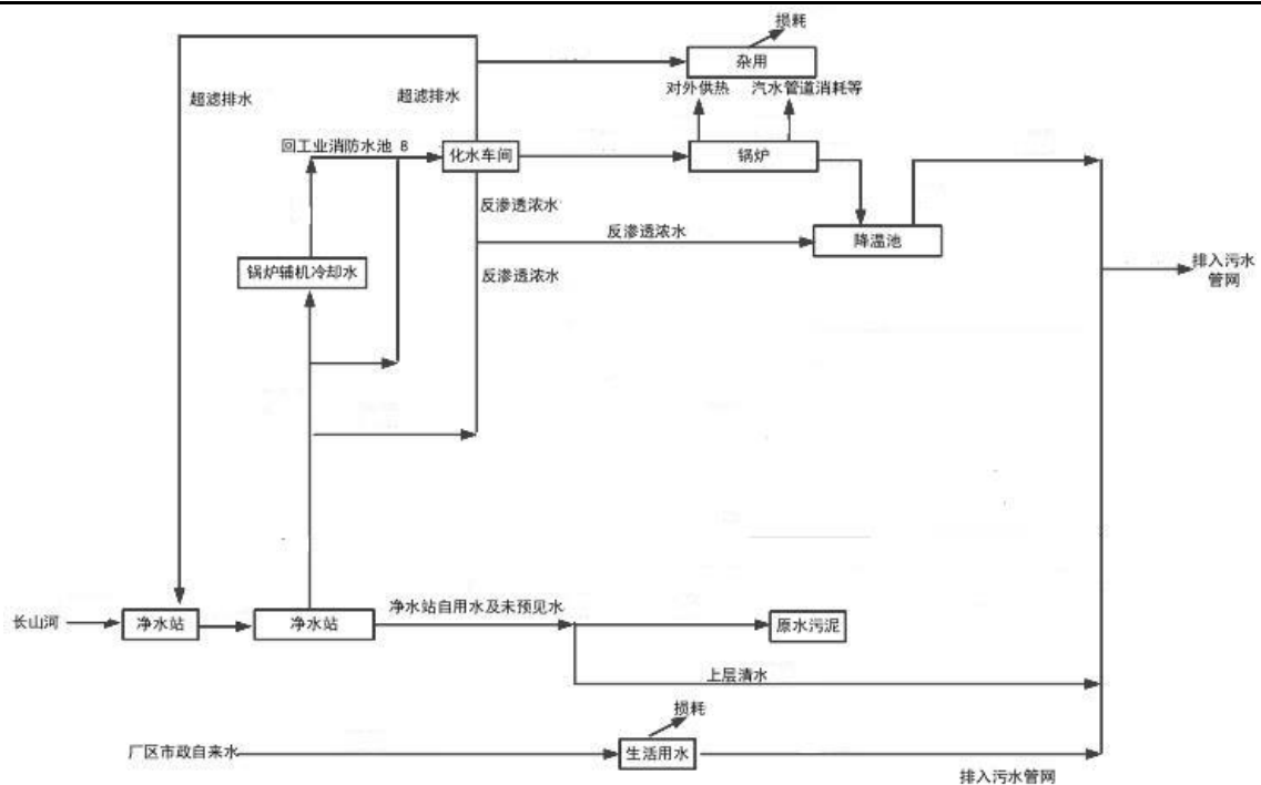
项目 2 号能源站水平衡图 单位: t/h
