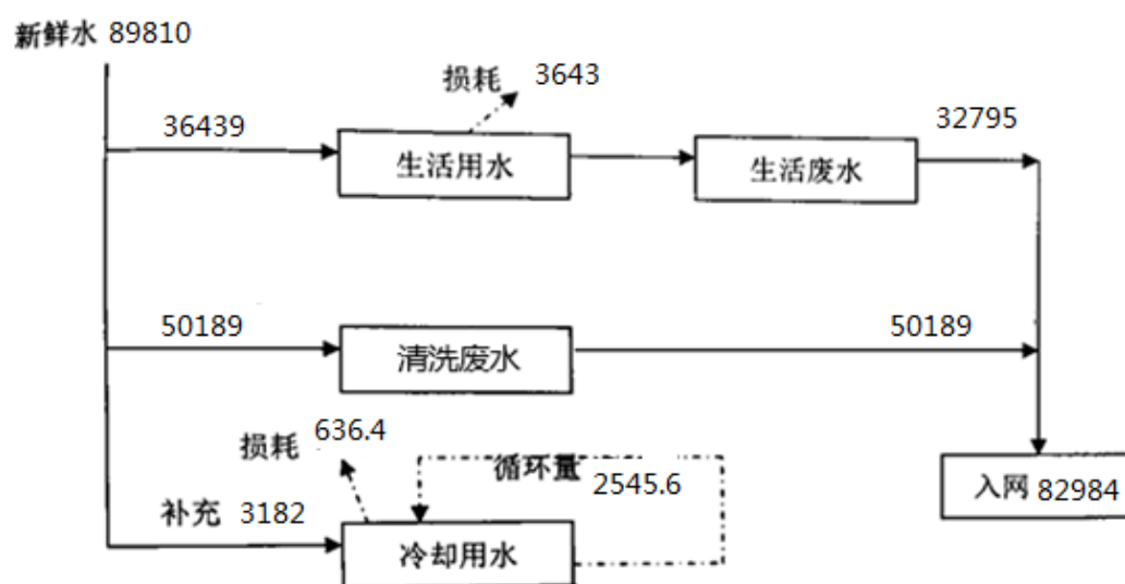
图 2-2 全厂水平衡图
