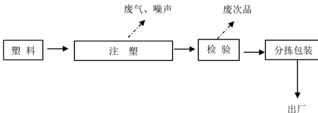
图 2-4 LED 塑料照明结构件生产工艺流程及产污位置图
