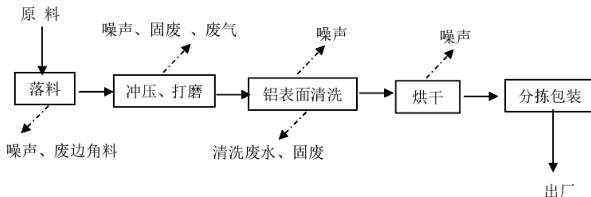
图 2-3 LED 金属照明结构件生产工艺流程及产污位置图
