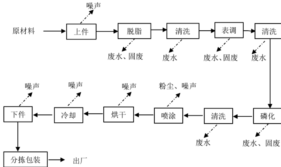
图 2-5 灯具金属件喷粉生产工艺流程及产污位置图
