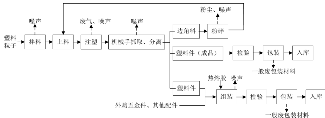
图 2-1 产品工艺流程及产污环节
