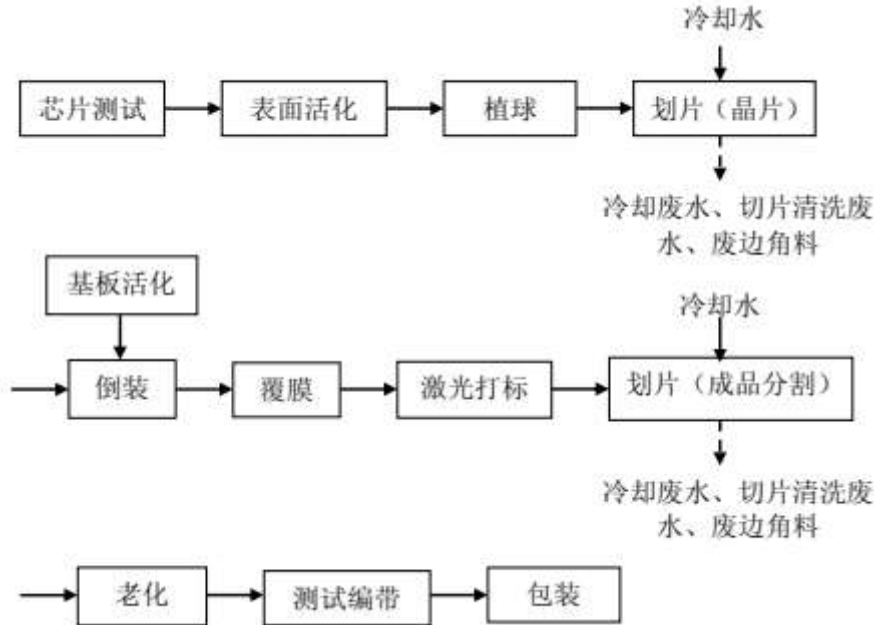
图 2-2 生产工艺流程及产污节点图
