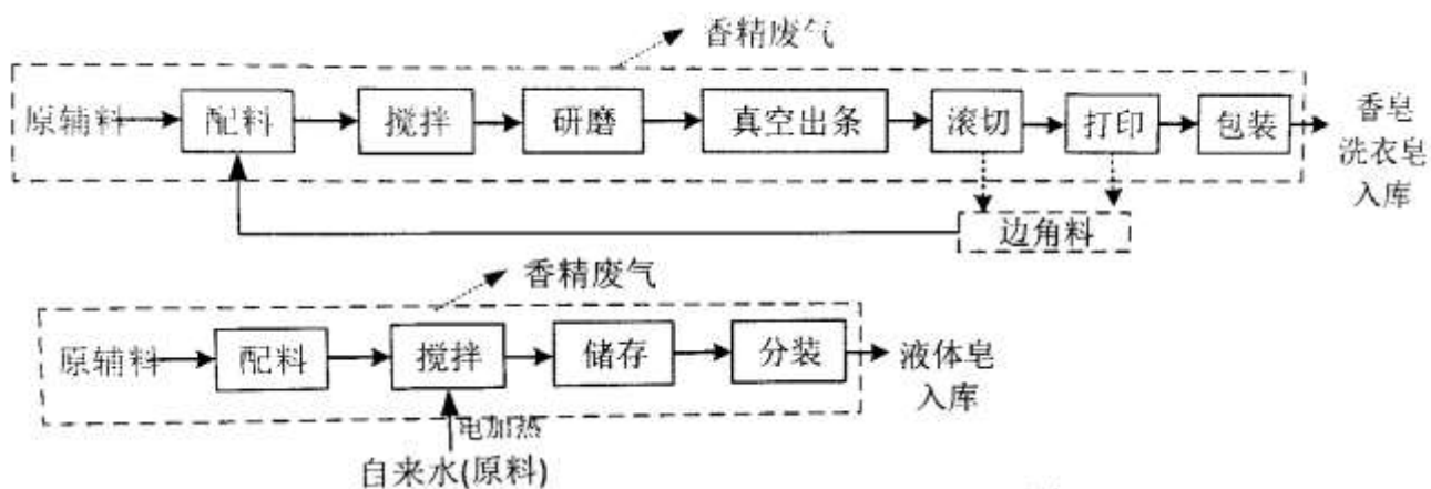
图 3-3 工艺流程及产污位置图
