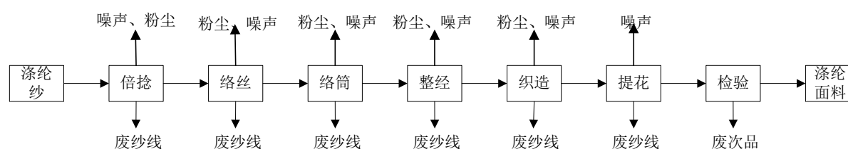
图 3-5 织造工序生产工艺流程图
