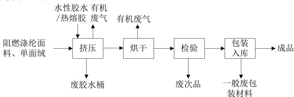
图 3-3 胶水复合工序生产工艺流程图
