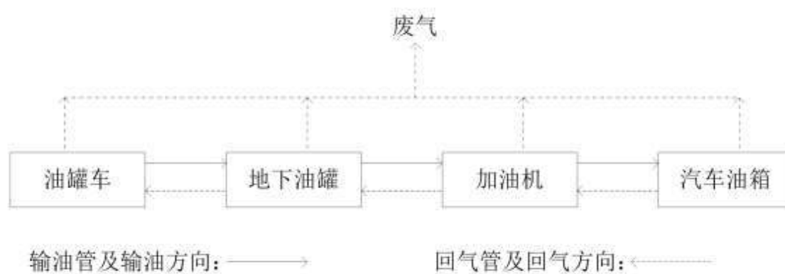
图 3-3 加油工艺及产污环节图
