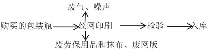
图 3-8 本技改项目包装瓶生产工艺流程及产污位置图
