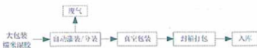
图 3-2 糯米湿胶分装工艺流程图
