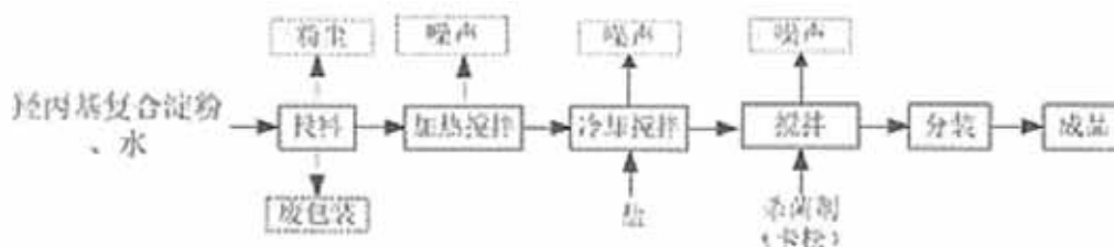
图 3-6 淀粉糯米湿胶生产工艺流程图
